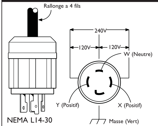
Figure 12 – Prise à Verrouillage de 120/240 Volts c.a., 30 Ampères
